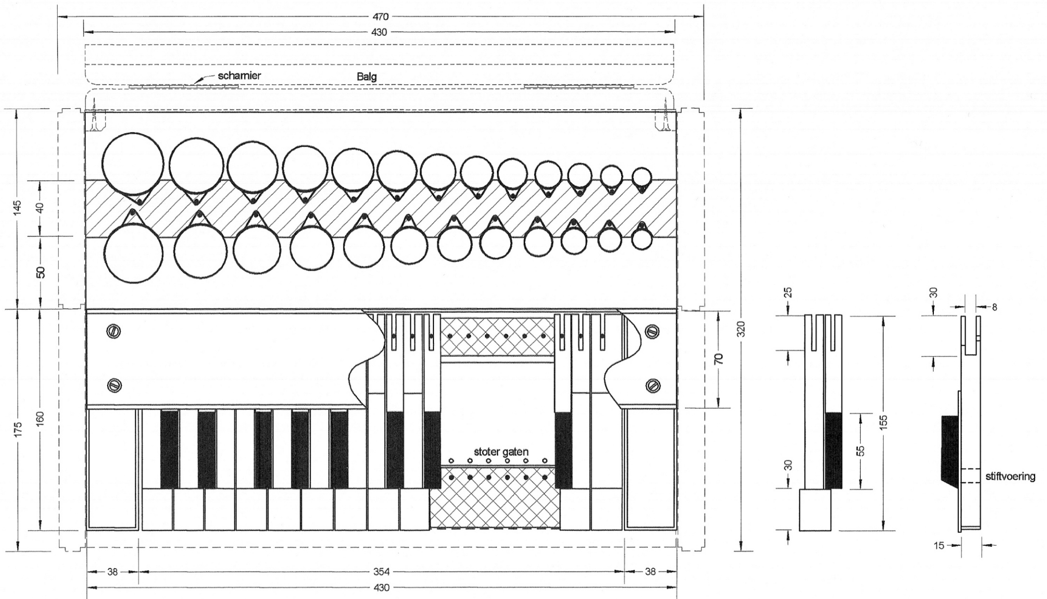
Tekening 2, bovenaanzicht windlade met klavier. De afdekbalk achter de toetsen is gedeeltelijk en een aantal toetsen zijn geheel weggelaten zodat de stotergaatjes, de stiften, het vilt, etc, zichtbaar zijn. Het gearcheerde deel tussen de pijpen geeft het plankje voor de pijpenhangers aan.
