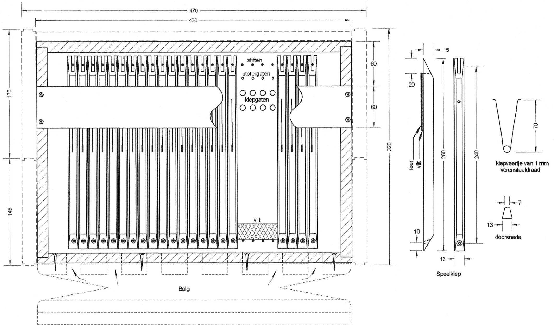
Tekening 7, onderaanzicht windlade zonder bodem. Een deel van het balkje waartegen de klepveren drukken is weggelaten zodat de kleppen zichtbaar worden. Een paar kleppen zijn weggelaten zodat de klepgaten, de stotergaatjes, vilt, etc. zichtbaar is. De doorvoergaten voor de wind van de balg naar de windlade zijn schematisch aangegeven.
