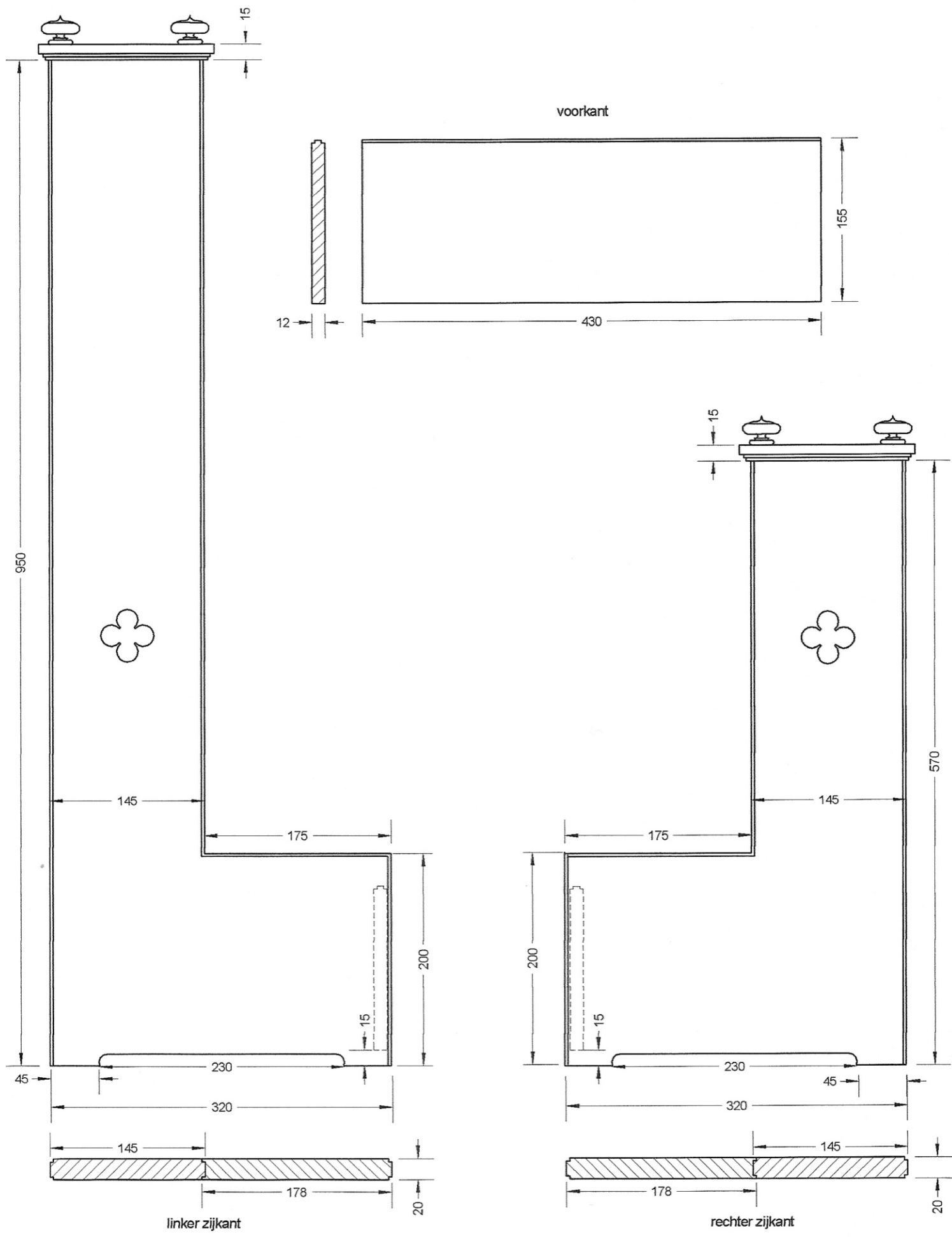
Tekening 10, de afzonderlijke kastdelen van het portatief. De zijkanten kunnen worden samengesteld uit twee delen. Alle sponningjes zijn 3x3 mm.
