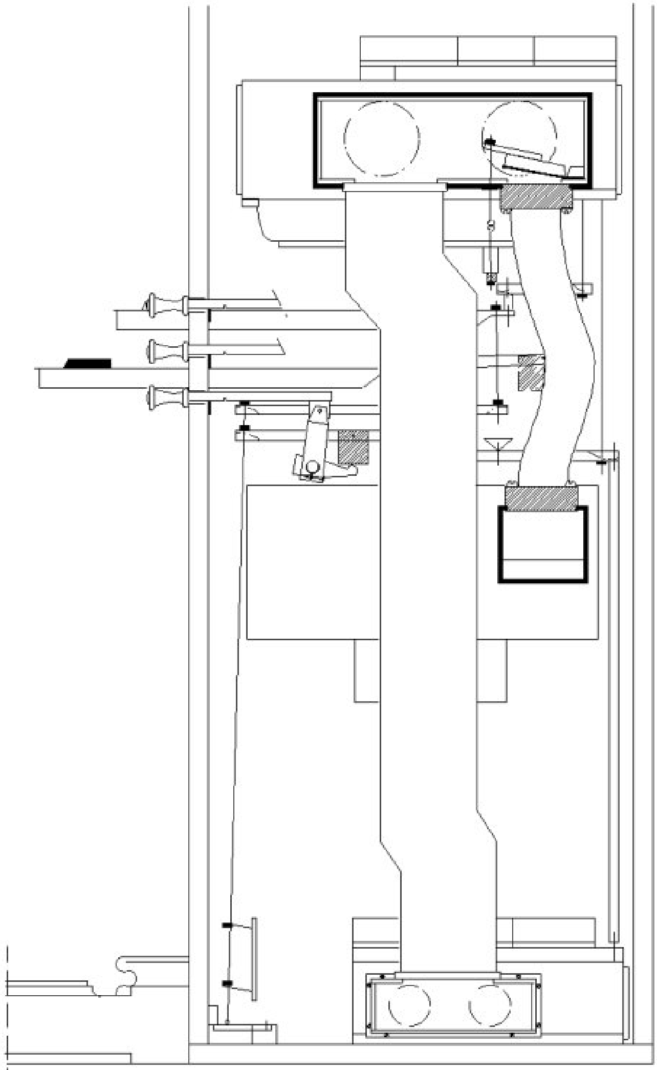
Zijaanzicht
